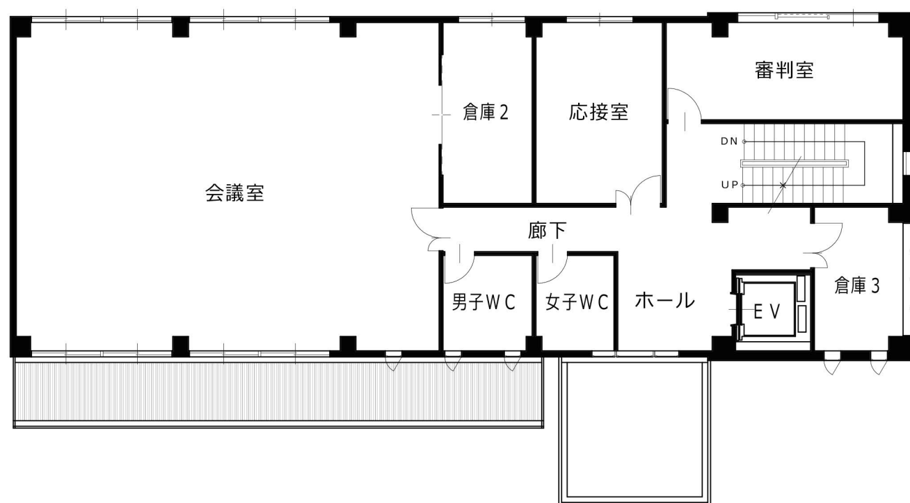
2階平面図
